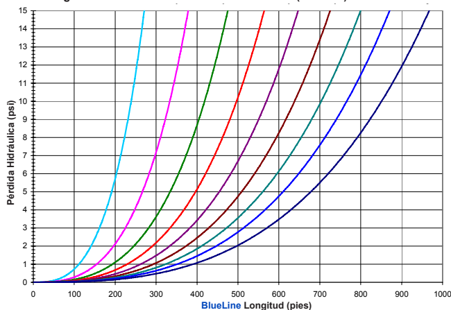
Pérdida Hidráulica vs. Longitud y Espaciamiento entre goteros: Manguera con Goteros BlueLine Classic de 18 mm (0.620" DI). Pendiente de 0%
