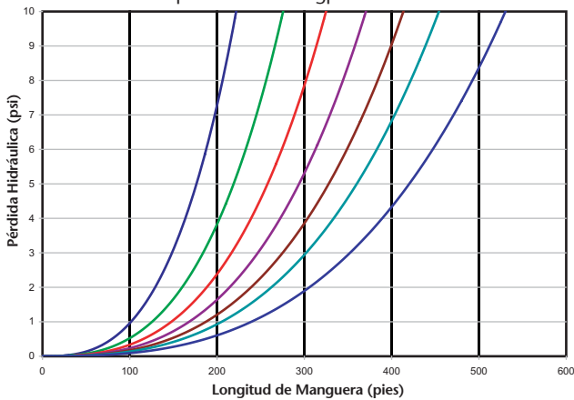
Pérdida de Carga Hidráulica vs. Longitud y Espaciamiento entre goteros: Gotero Drip In Classic 1.08 gph. Pendiente de 0%
