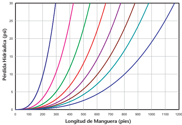
Pérdida Hidráulica vs. Longitud y Espaciamiento entre goteros: Gotero Drip In PC 0.63 gph. Pendiente de 0%
