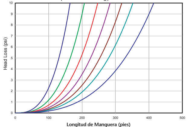
Pérdida de Carga Hidráulica vs. Longitud y Espaciamiento entre goteros: Gotero Drip In Classic 1.8 gph. Pendiente de 0%
