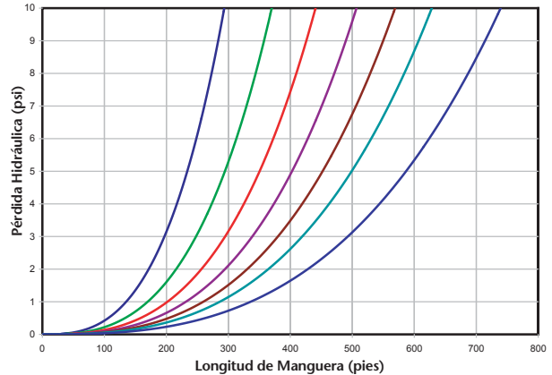
Pérdida de Carga Hidráulica vs. Longitud y Espaciamiento entre goteros: Gotero Drip In Classic 0.75 gph. Pendiente de 0%
