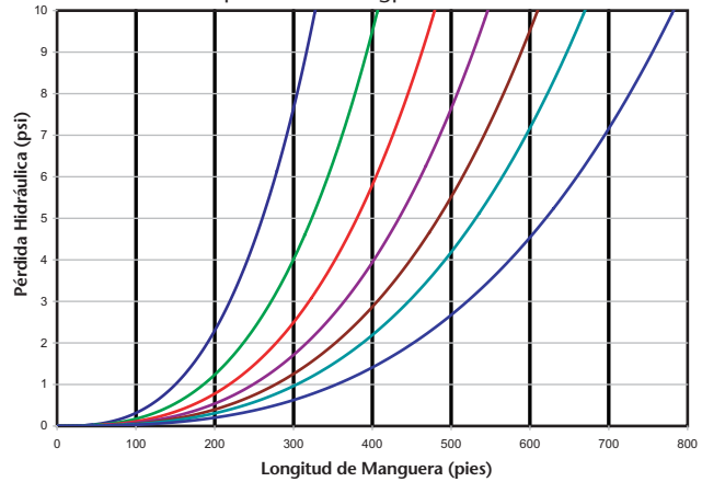
Pérdida de Carga Hidráulica vs. Longitud y Espaciamiento entre goteros: Gotero Drip In Classic 1.0 gph. Pendiente de 0%
